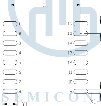
图 18. 16 引脚宽体 SOIC 封装 [WB SOIC-16] 焊盘图案
