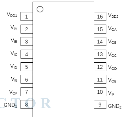
图 4.π161Uxx 管脚定义
