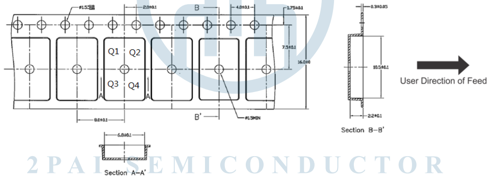
图 200. 16 引脚窄体 SOIC 封装 [NB SOIC-16] 包装信息-尺寸单位(mm)
