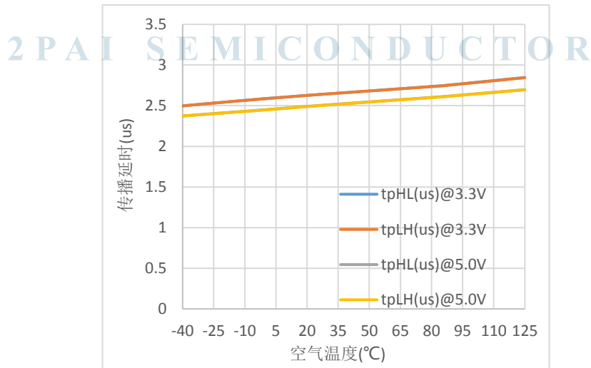
图 10.π16xU6x 传输延时 vs. 空气温度
