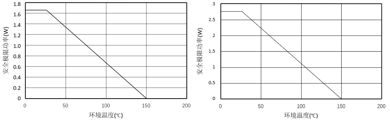
图 7.热降额曲线, 依据 DIN V VDE V 0884-11 的安全限值与环境温度的关系(左: π16xU3x; 右: π16xU6x)
